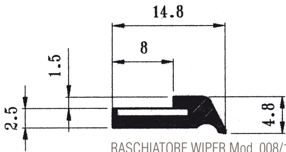
RASCHIATORE WIPER Mod. 008/11109 Materiale Acciaio-NBR Material Steel-NBR In barre / Bars Length 560 mm
