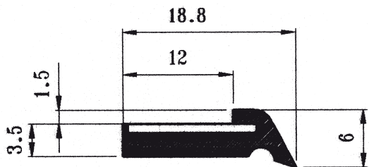
RASCHIATORE WIPER Mod. 008/11110 Materiale Acciaio-NBR Material Steel-NBR In barre / Bars Length 560 mm
